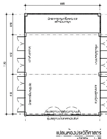
ภาพ 1 แผนผังแสดงแปลน (plan) โดยรวมการแบ่งพื้นที่การจัดแสดงภายในห้องประวัติศาสตร์ศูนย์วัฒนธรรม
