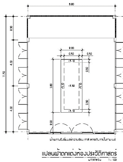
ภาพ 3 แผนผังแสดงแปลน (plan) แบบฝ้าเพดานพื้นที่การจัดแสดง ภายในห้องประวัติศาสตร์ศูนย์วัฒนธรรม
